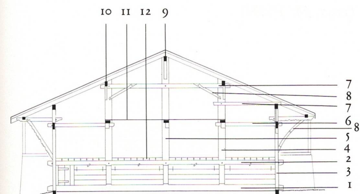
919 Coupe transversale A-A 1:200
