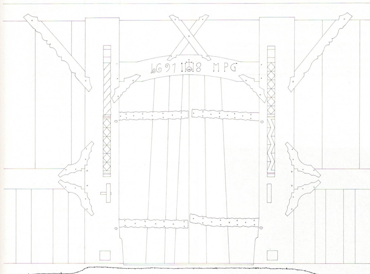
921 Porte de grange 1:50
